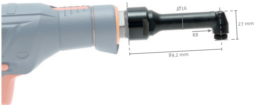
Der Bit wird mit einem Sicherungsring und Überwutmutter aufgenommen 1/4" internal hex with locking ring and coupling nut
