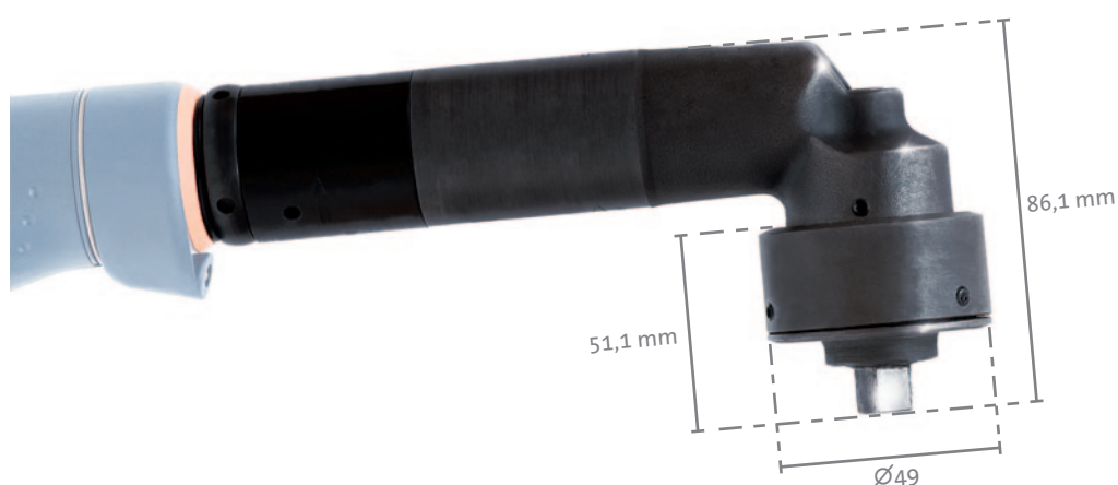
Lieferbar mit 3/8 Avkt. und 1/2" Avkt. Available with 3/8 square and 1/2" square
